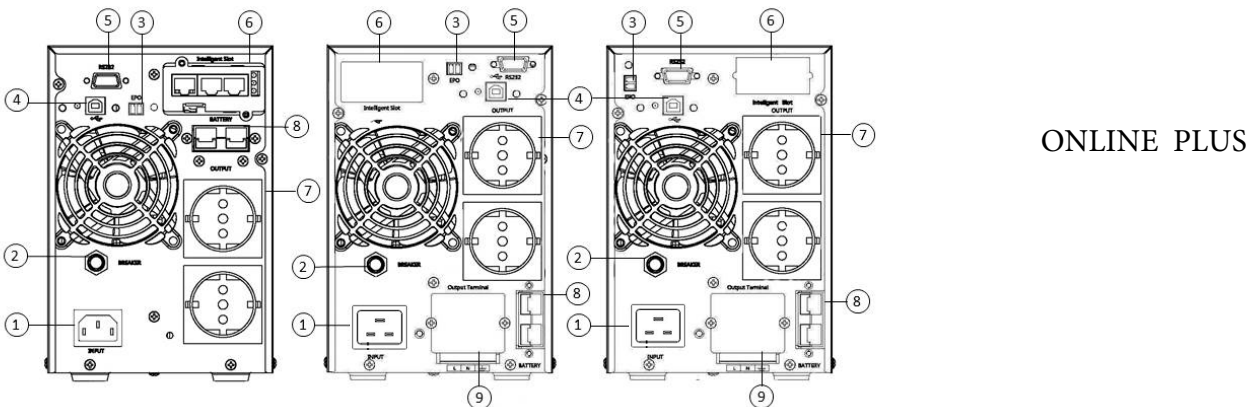
Рис.3 Задняя панель ИБП серии ONLINE PLUS 1000/2000/3000.
