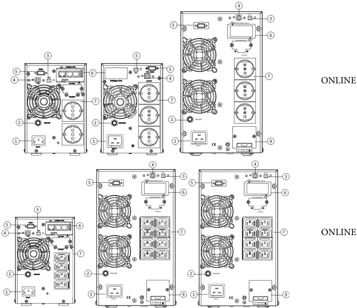
Рис.2 Задняя панель ИБП серии ONLINE и ONLINE I 1000/2000/3000.
