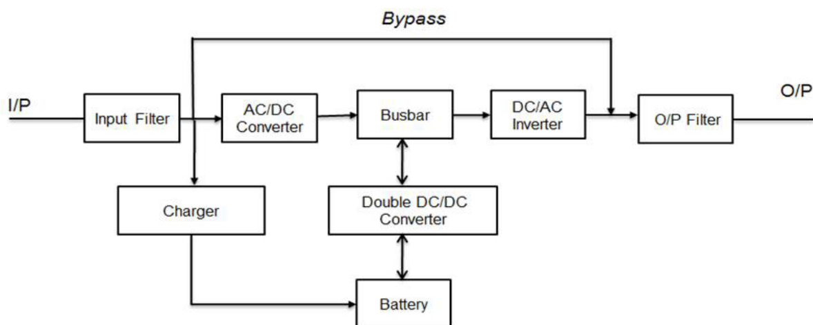
Рис.1 Блок-схема ИБП
