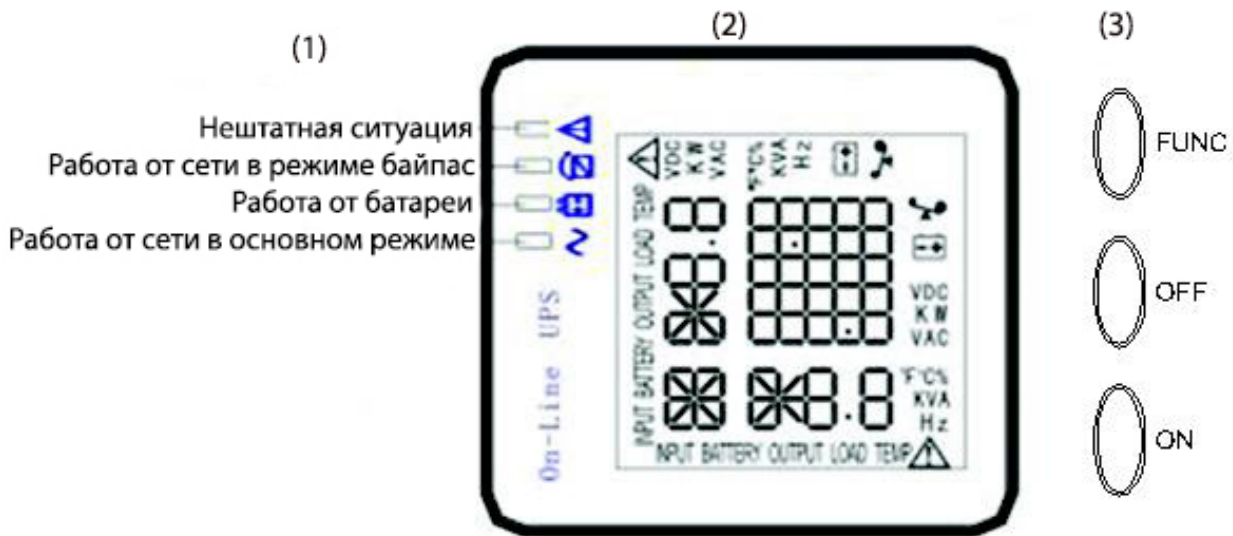
Рис. 4. Панель управления ИБП
