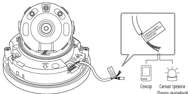
<QNV-6010R/6020R/6030R>
